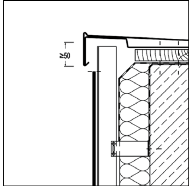
PARAPETAS (vertikalus pjūvis)
