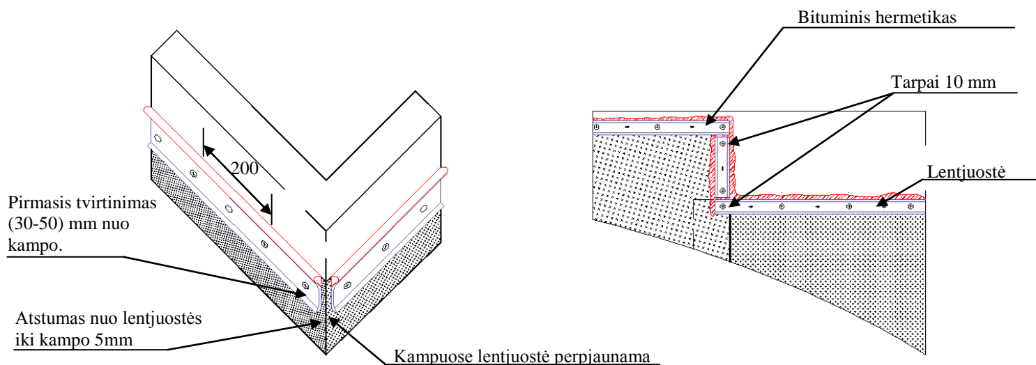
42 pav. Lentjuostės montavimas dangos kampe. 43 pav. Dangos krašto apipavidalinimas lentjuoste
