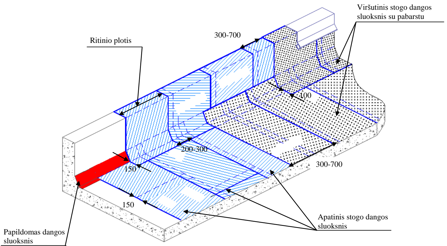
50 pav. Ritininių dangų išdėstymas sudūrimo su parapetu vietose. 2 variantas.
