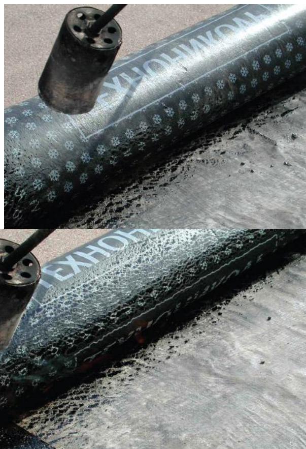
34 pav. Piešinio dingimas apatinėje ritinio pusėje, teisingai kaitinant paviršių.
