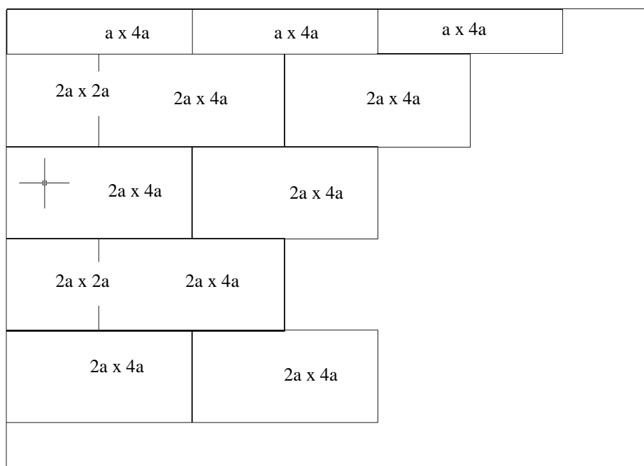
21 pav. Pirmojo termoizoliacinio sluoksnio klojimo schema
