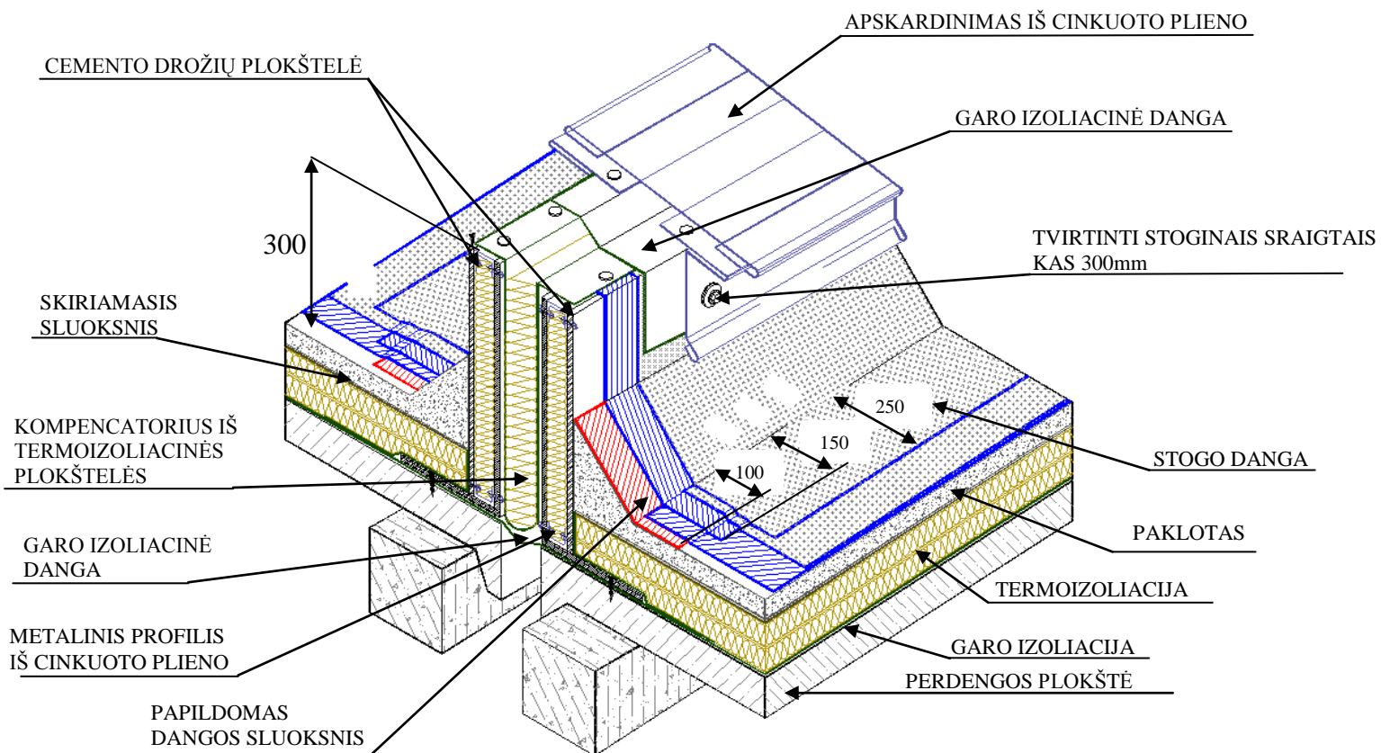
14 pav. Deformacinė siūlė
