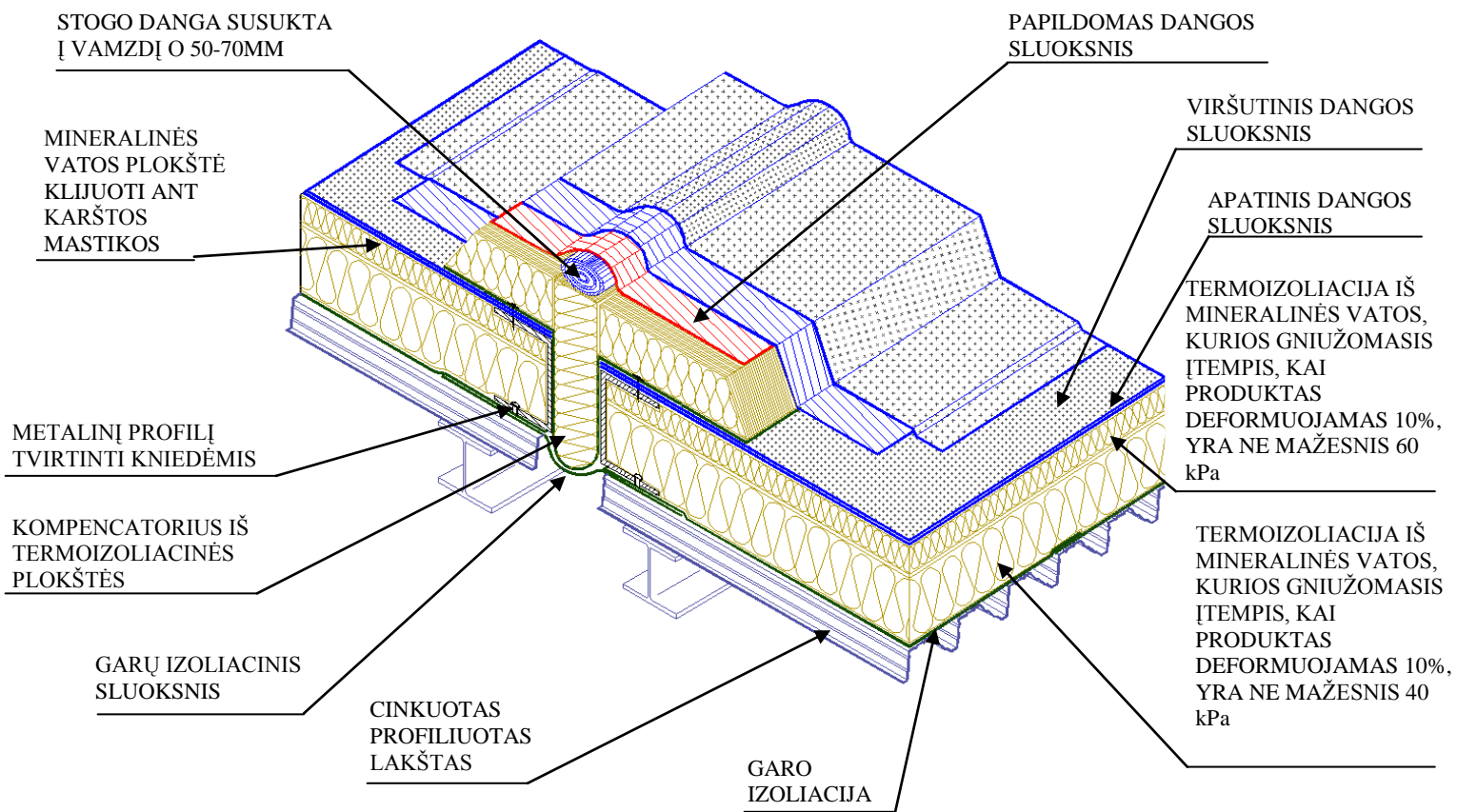
16 pav. Deformacinė siūlė dangose su pagrindu iš profiliuoto lakšto.
