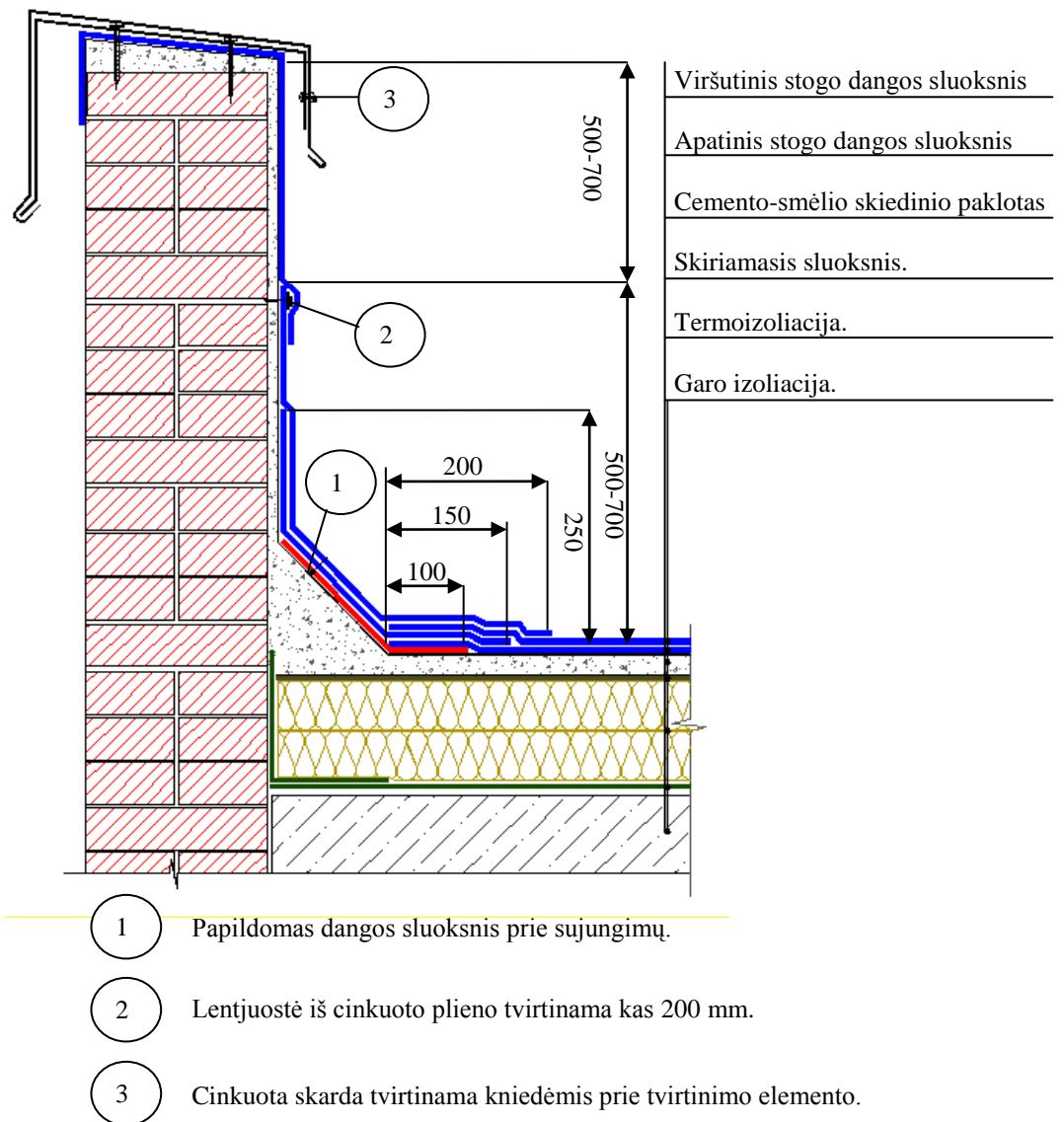
51 pav. Stogo dangos prijungimas prie aukštos parapetinės sienos.
