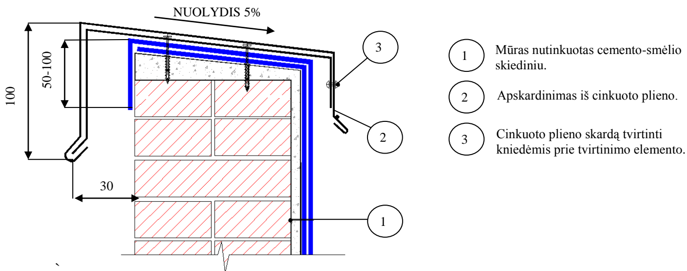
47 pav. Stogo dangos sujungimas su parapeto siena, žemesne nei 500 mm.
