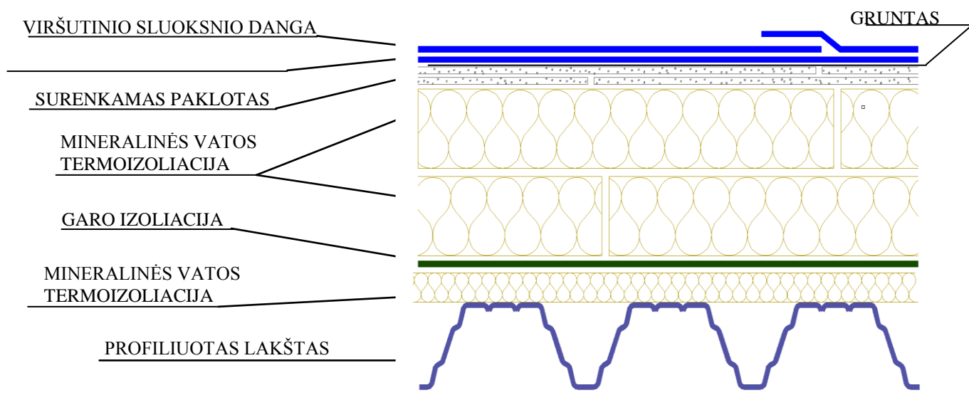
8 pav. Surenkamieji išlyginamieji paklotai
