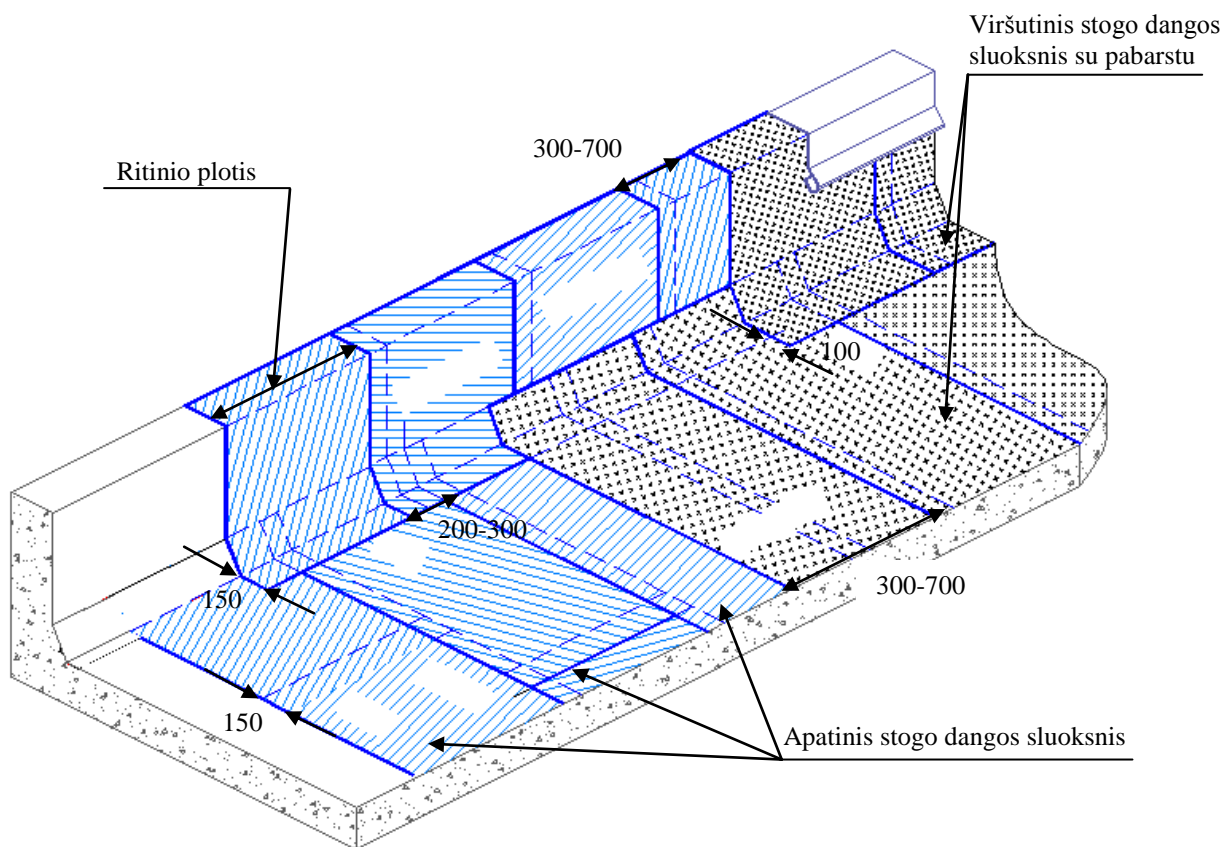
48 pav. Stogo dangos sujungimas su parapetu .
