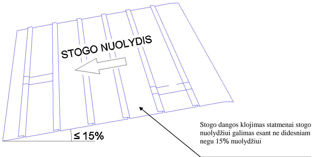
29 pav. Dengimas danga ant šl:
