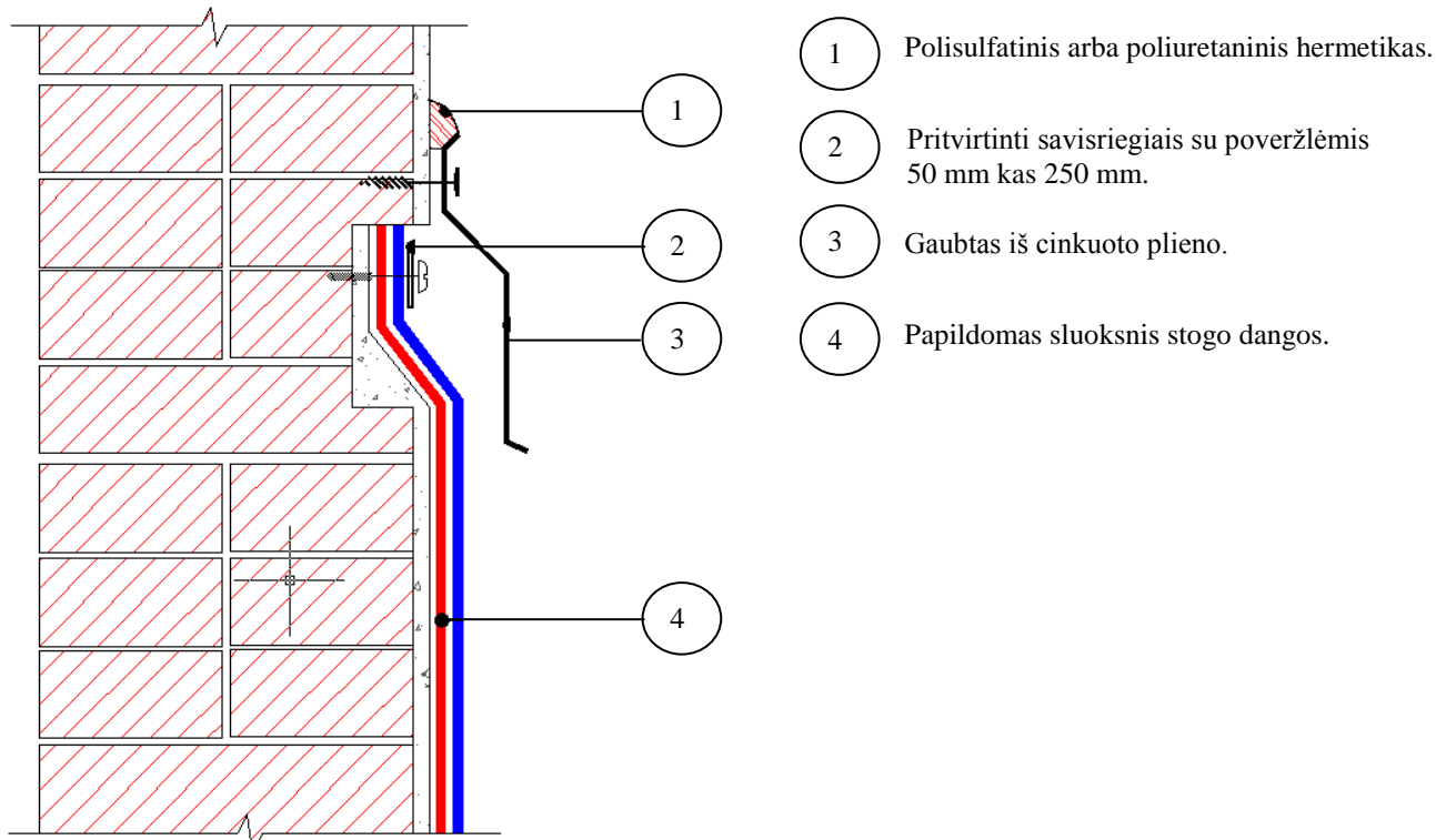
45 pav. Stogo dangos krašto sujungimas parapeto sienos lovyje.
