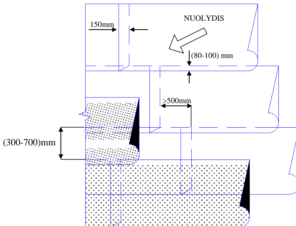
32 pav. Poslinkis sutampančiose stogo dangų sluoksniuose
