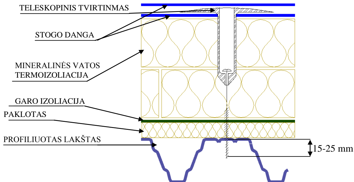
24 pav. Teleskopinis tvirtinimas.
