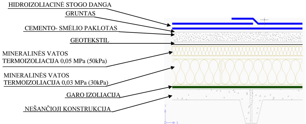
2 pav. Paklotas - gelžbetonio plokštės arba cemento smėlio denginys
