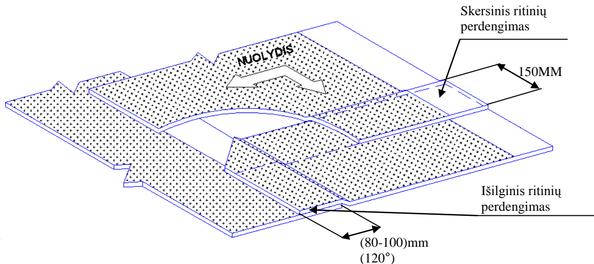
30 pav. Ritinių dangų perdengimas
