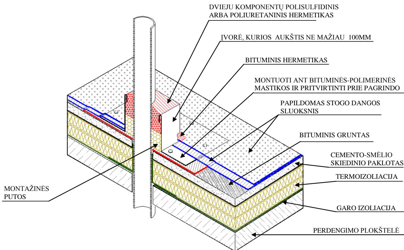
13 pav. Stogo dangos prijungimas prie mažo diametro vamzdžių ar vamzdžių pluošto.
