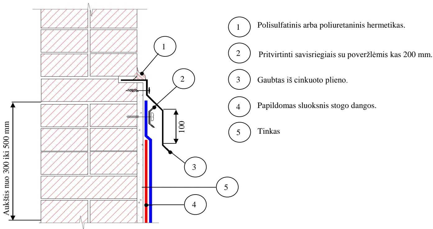
46 pav. Stogo dangos krašto sujungimas su plytine siena.
