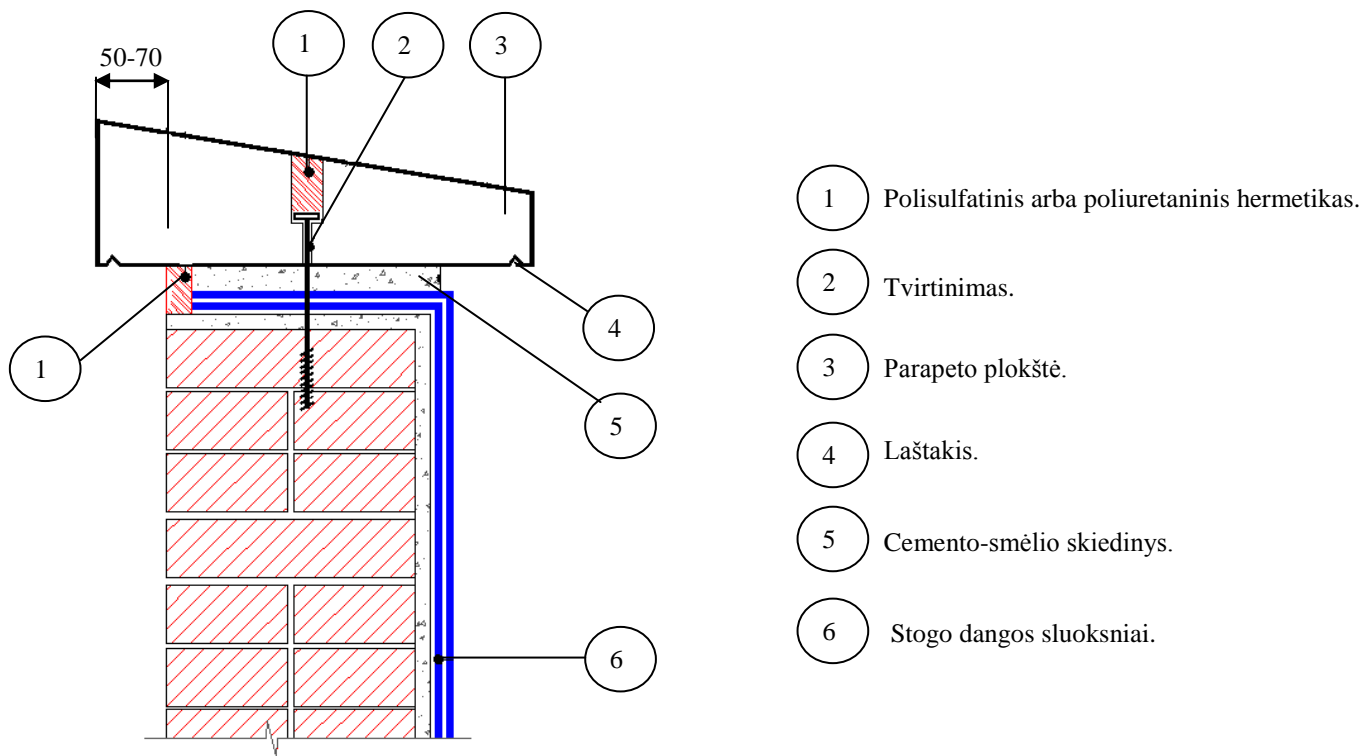
48 pav. Stogo dangos sujungimas su parapetu .
