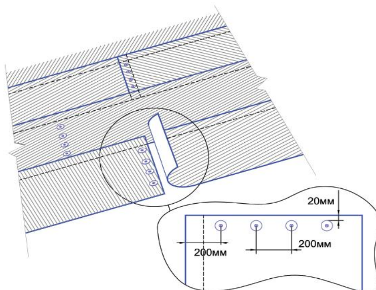
9 pav. Ritinio vidurio fiksavimas.
