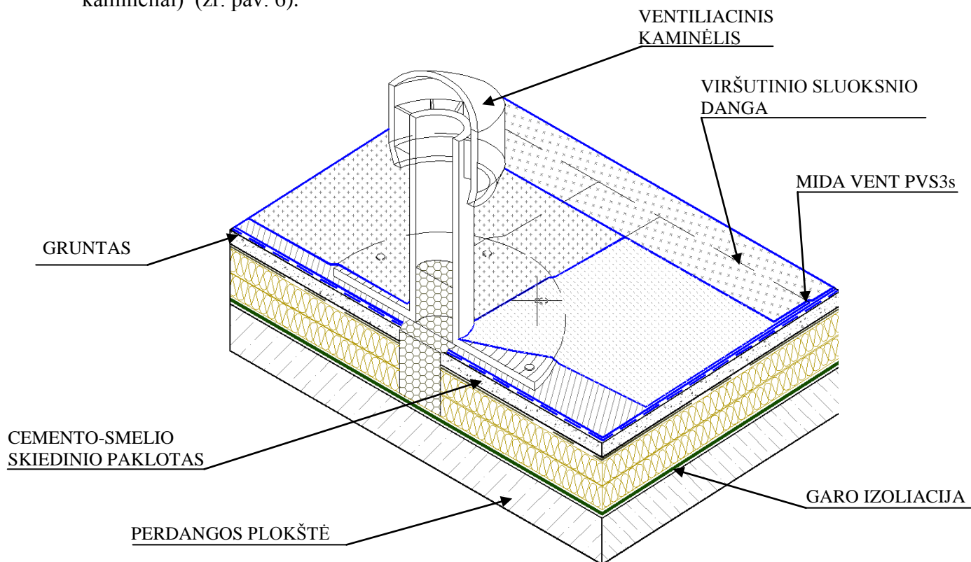
6 pav. Ventiliacinis kaminėlis
