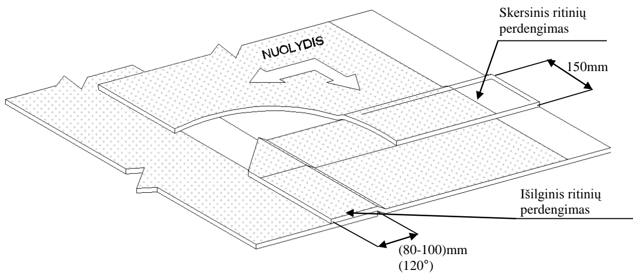
31 pav. Ritinių dangų perdengimas tvirtinant medžiagas mechanškai
