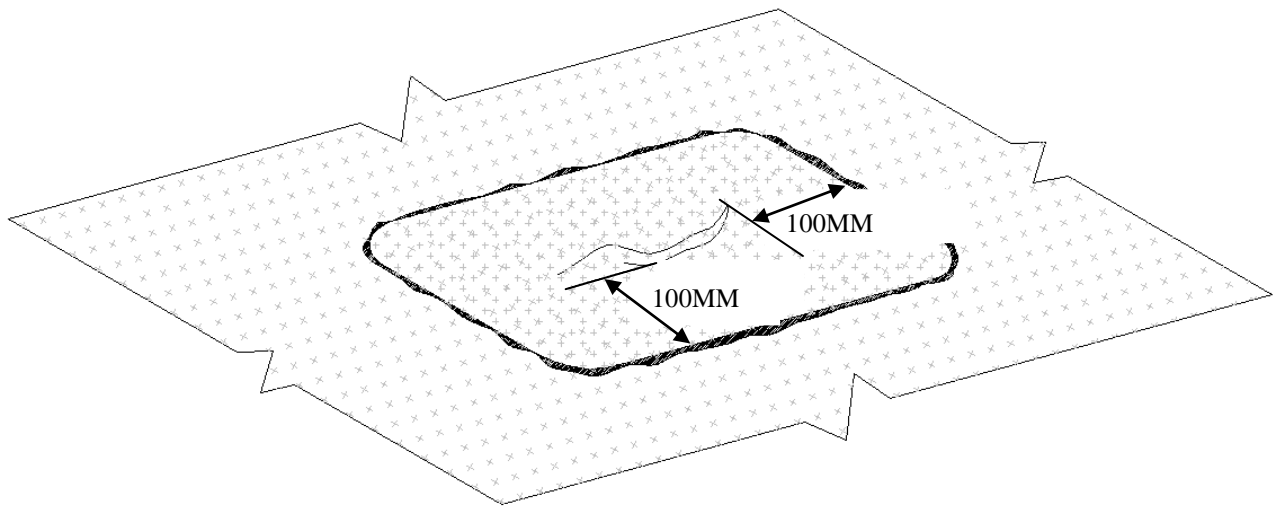
52 pav. Stogo dangos remontas, esant mechaniniam pažeidimui
