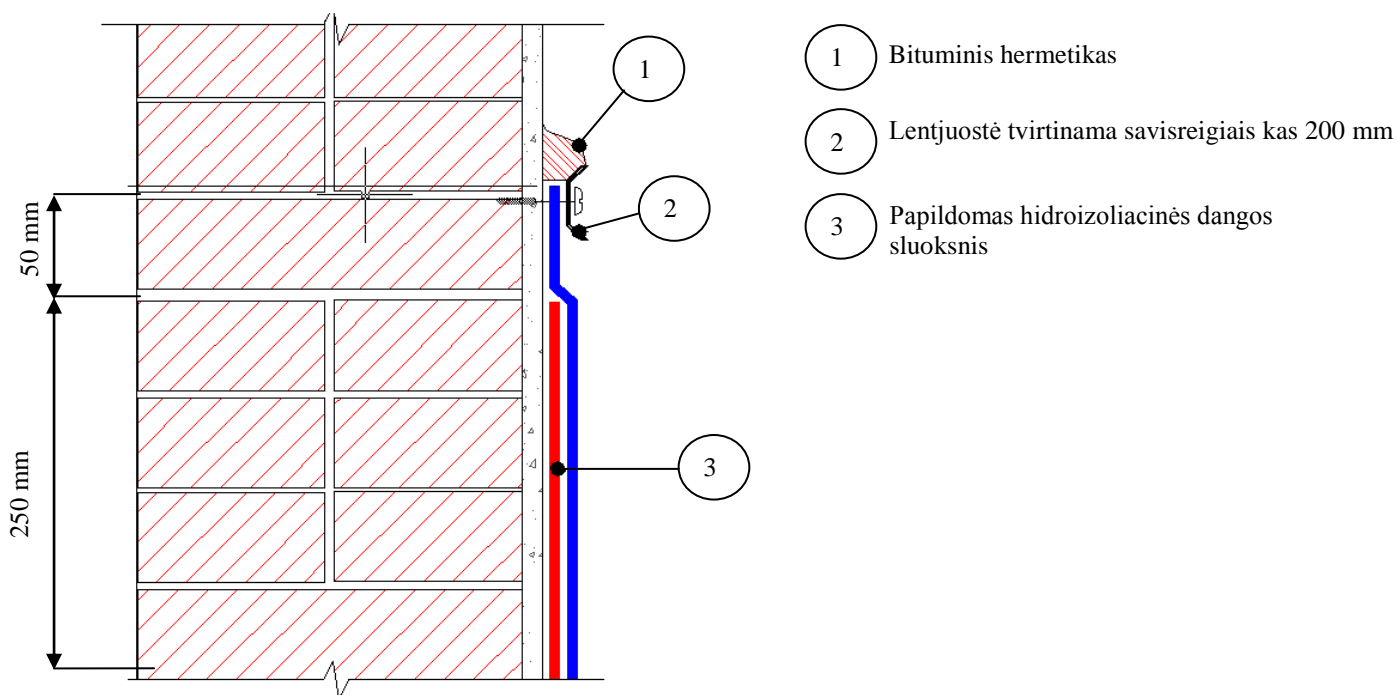
41 pav. Stogo dangos krašto pritvirtinimas lentjuoste (metaline juosta)
