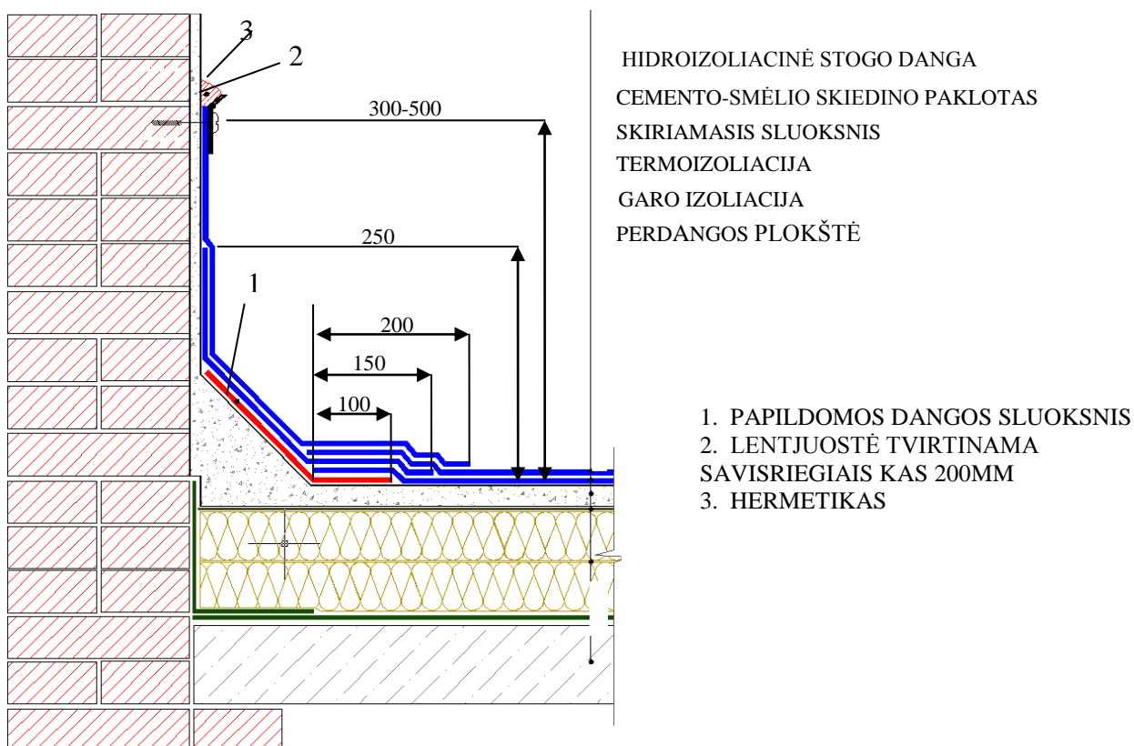
10 pav. Pagrindiniai stogo dangos sluoksniai ir papildomi sustiprinimo sluoksniai stogo dangos sujungimo su išsikišančiais virš stogo dangos elementais (parapeto siena)
