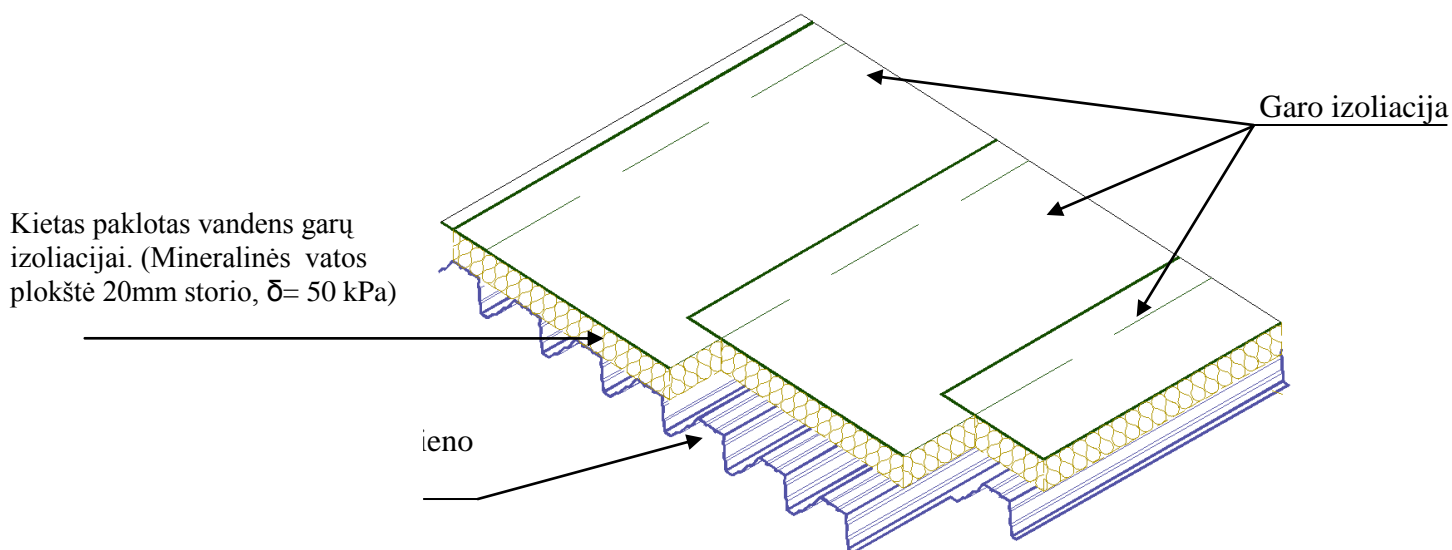
18 pav. Garų izoliacijos sluoksnio įrengimas ant profiliuoto lakšto
