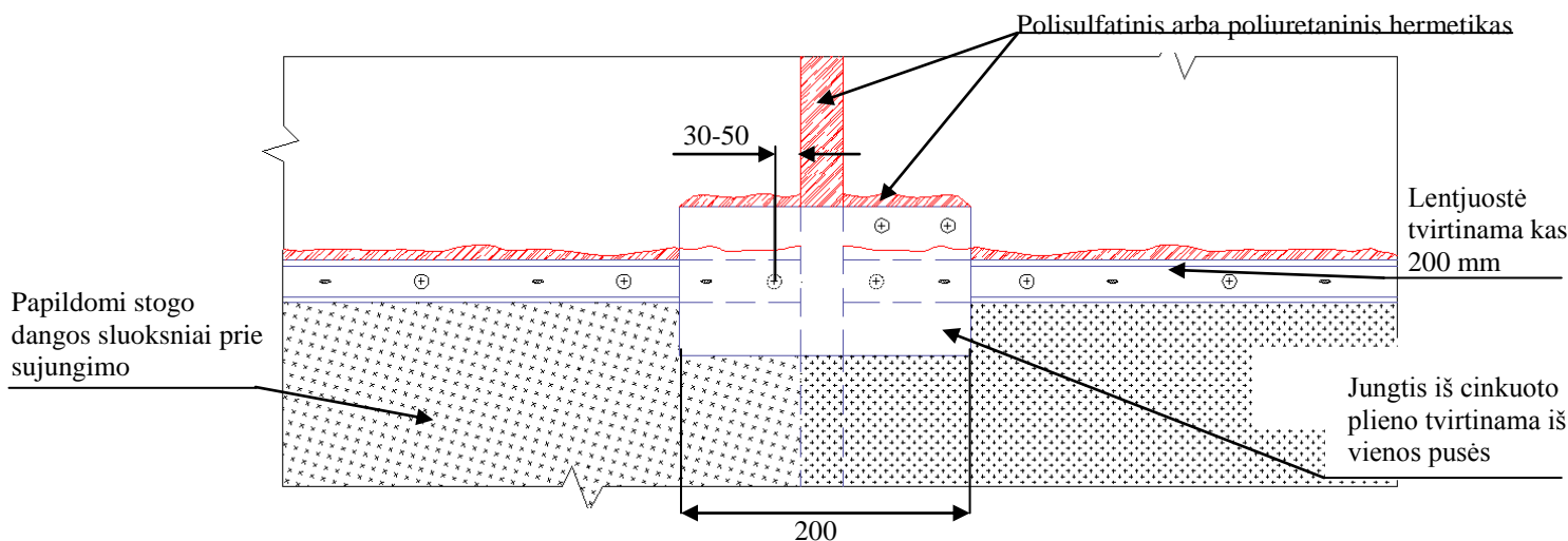
44 pav. Kraštinė juosta ant sienos iš betoninių plokščių.
