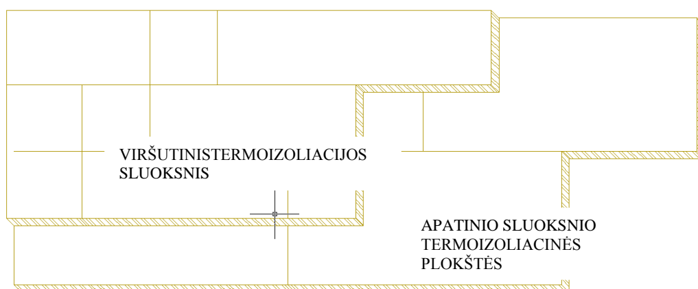
19 pav. Termoizoliacinių plokščių slinktis klojant viršutinį ir apatinį sluoksnius.
